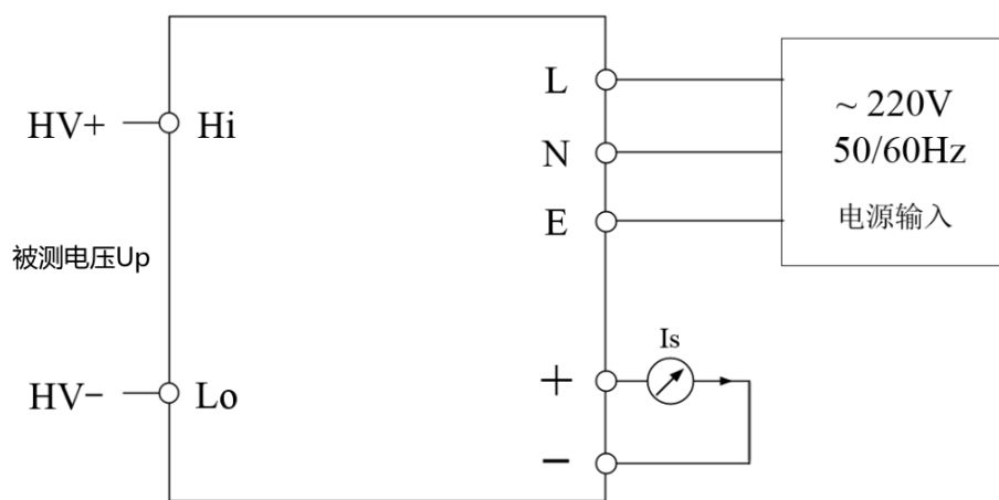
图 4 电气连接图
