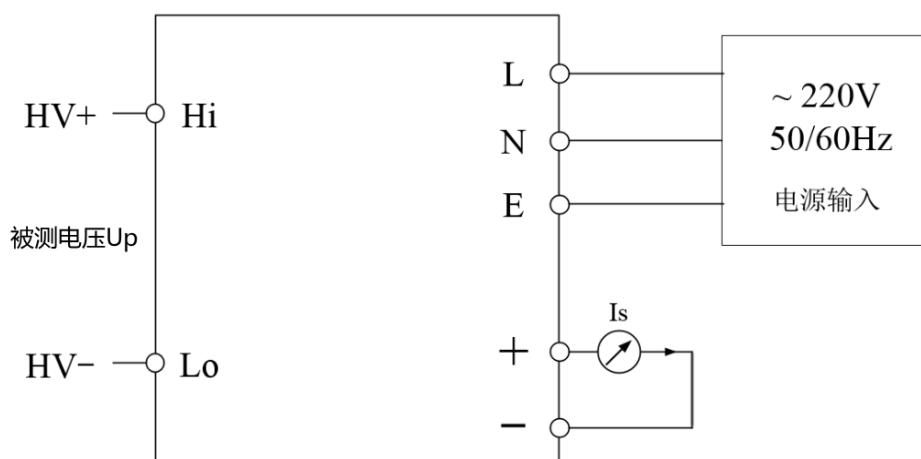
图 4 电气连接图
