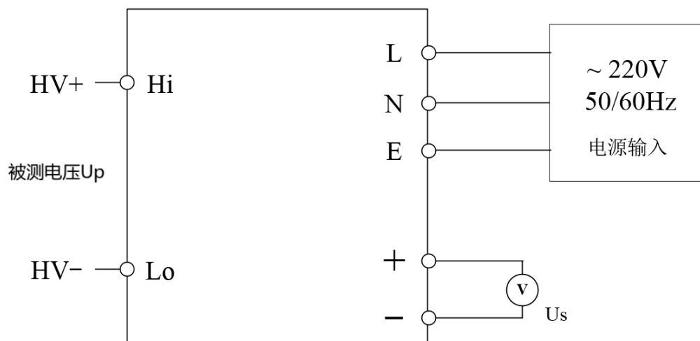
图 4 电气连接图
