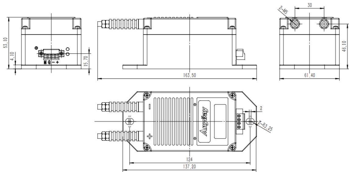
图 1 外形尺寸图
