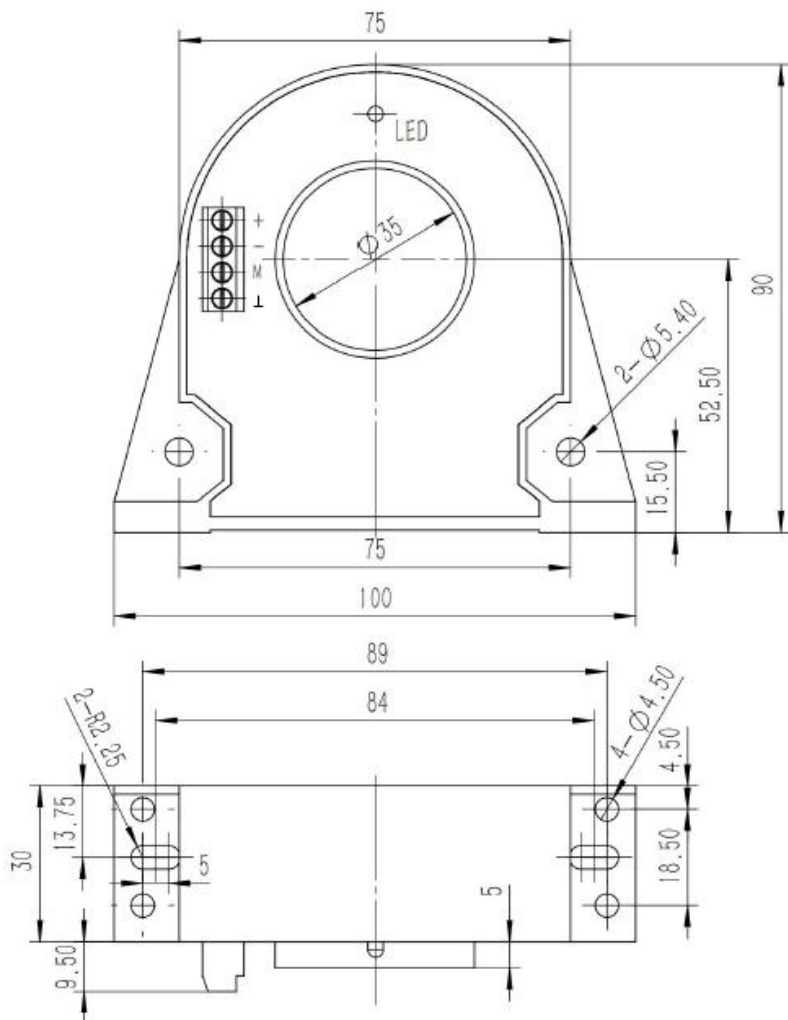
图 1 外形图
