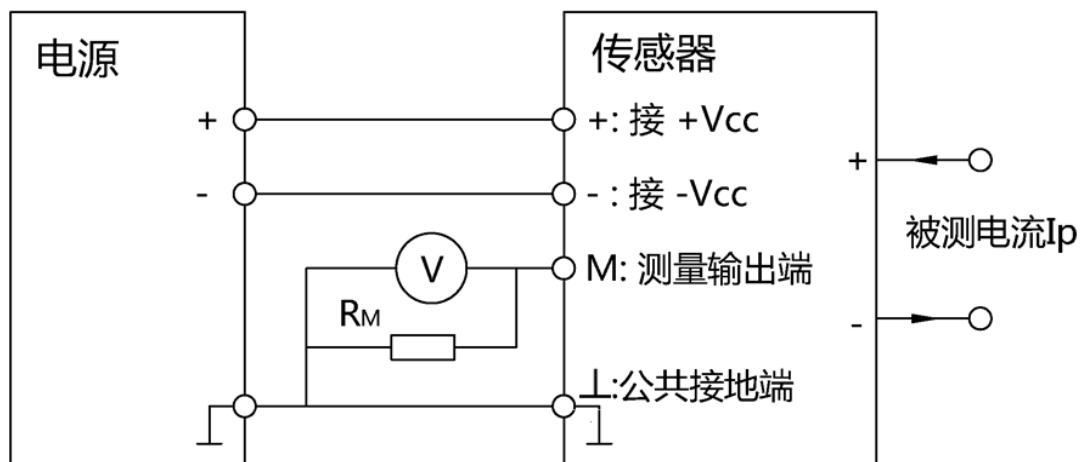
电气连接图
