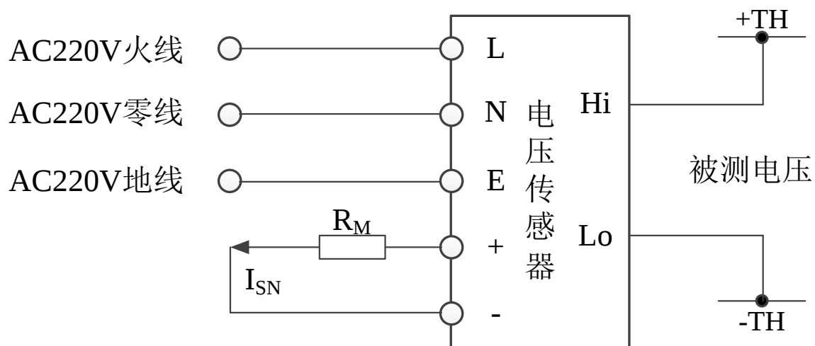
图3 电气连接图
