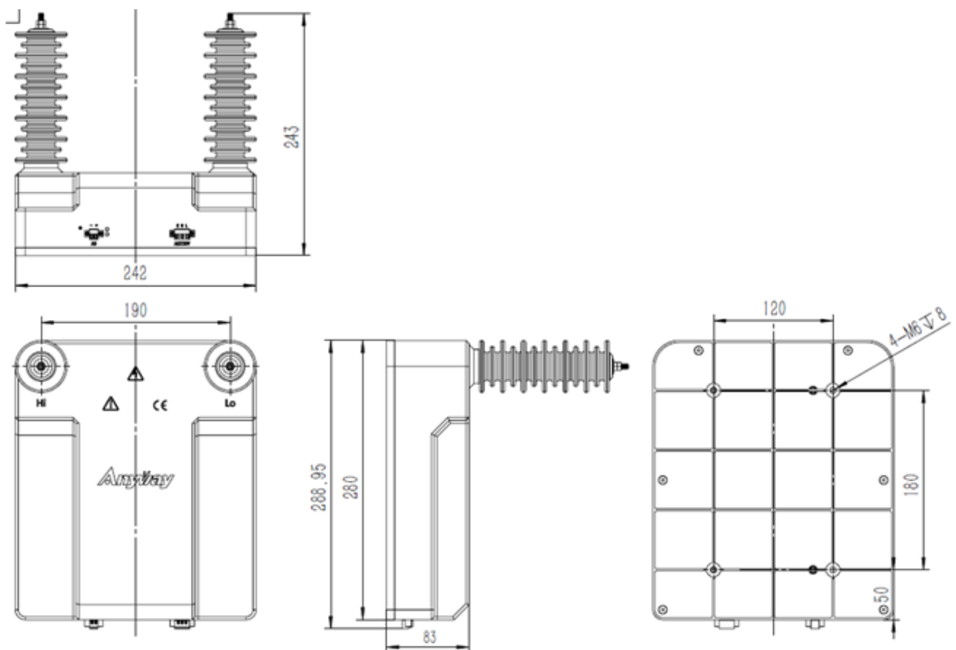
图 1 外形尺寸图
