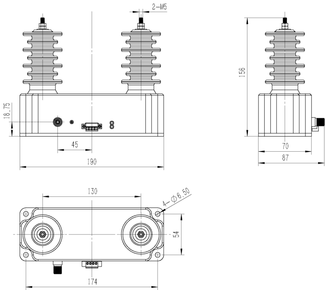
图 1 外形尺寸图
