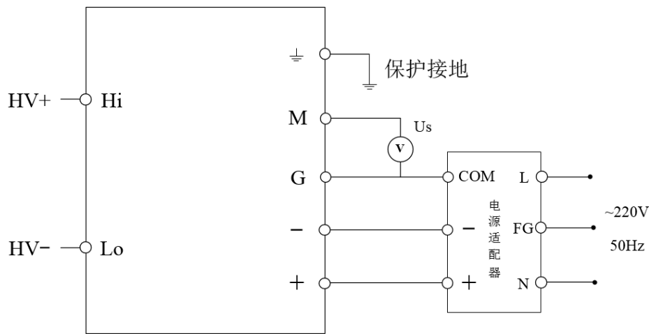
图 3 电气连接图
