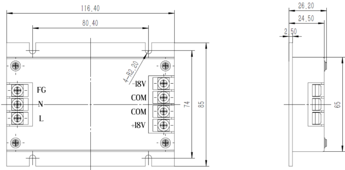
图 2 电源外形尺寸图
