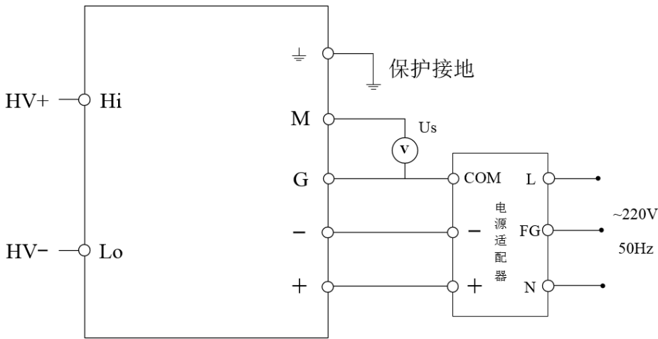
图 3 电气连接图
