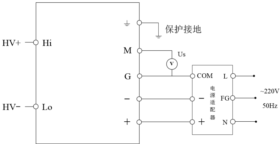
图 3 电气连接图
